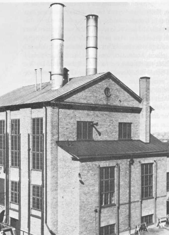
Ångcentralen — nu riv- ven — valdes som plats för Linköpings reläsän- dare. Mellan centralens skorsten och en 25 me- ter hög trämast, spän- des antennen, som var 20 meter lång.
